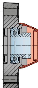
Ghiera eccentrica Locking collar Exzenter-Klemmring
